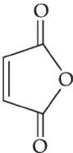
Maleic anhydride
